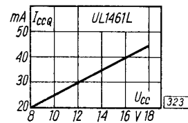
Prąd spoczynkowy zasilania w funkcji napięcia zasilania
